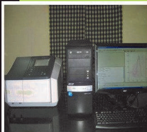
UV-VIS
